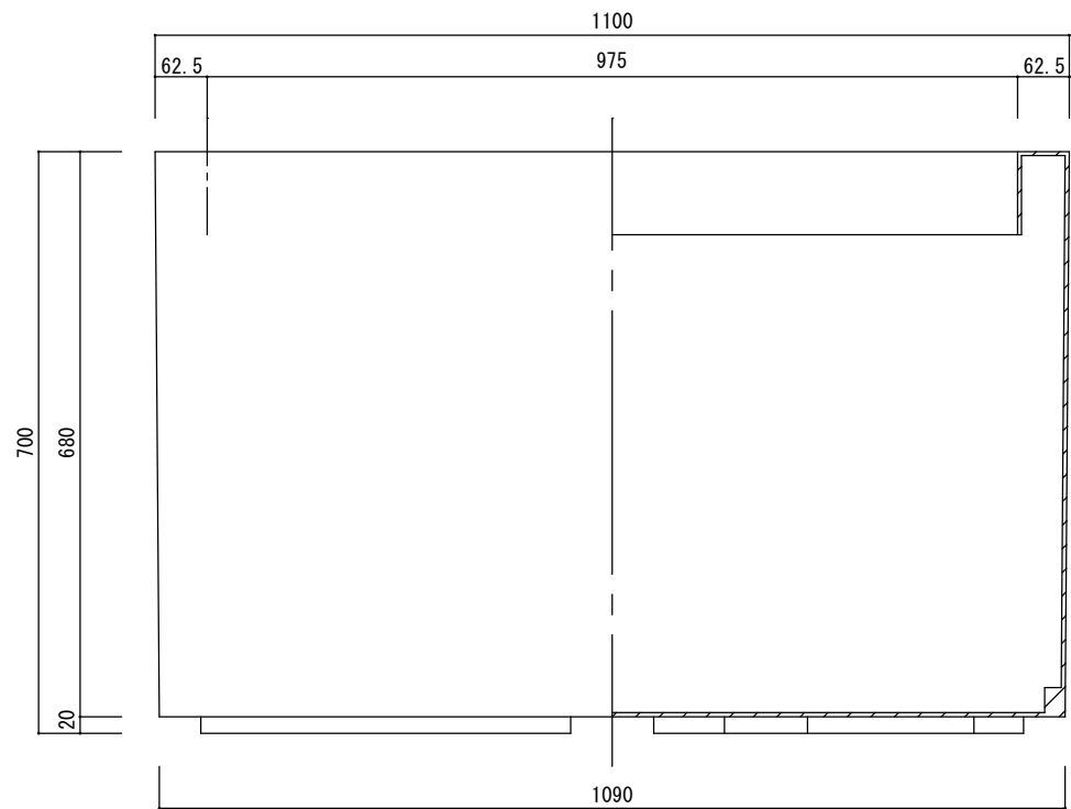
立・断面図
