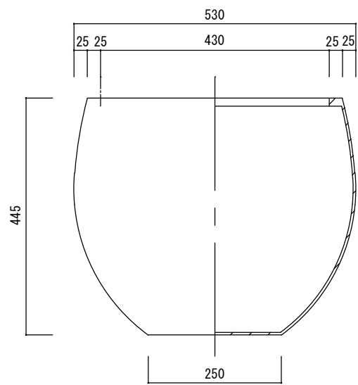
立・断面図
