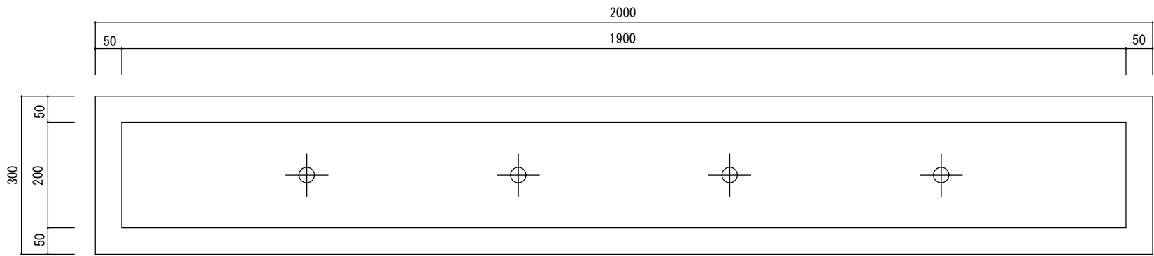
平面図
