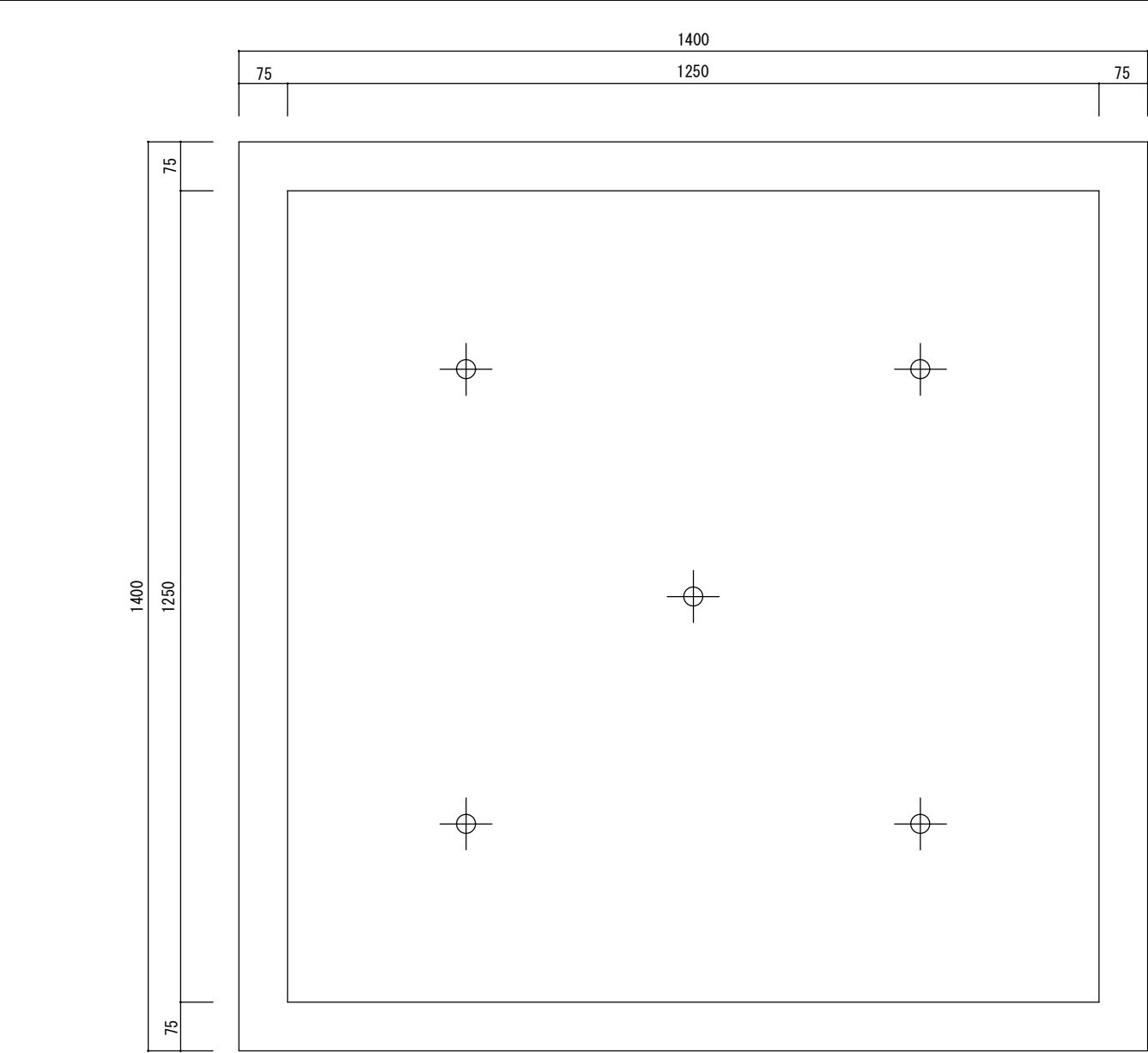
平面図
