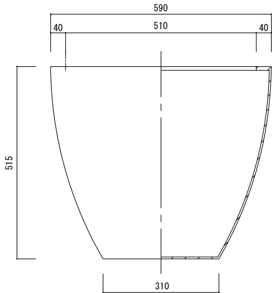
立・断面図
