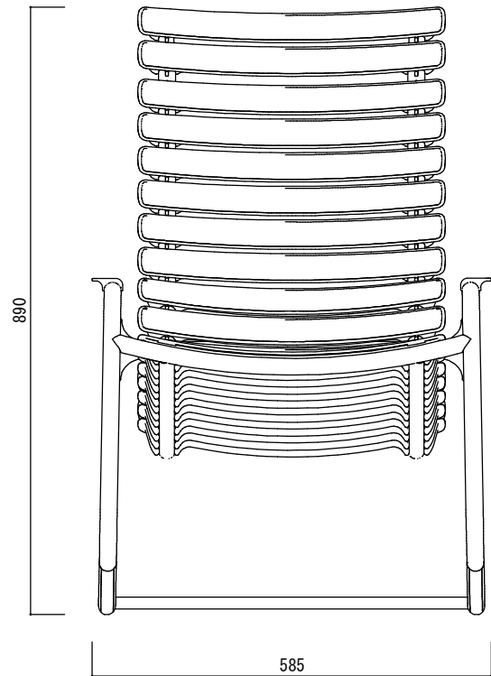
立面図
