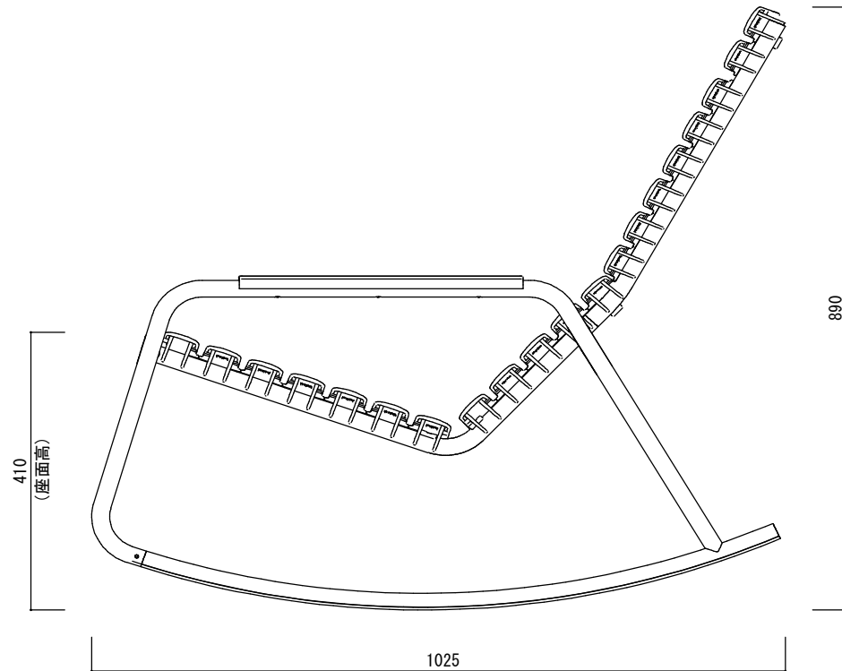
側面図
