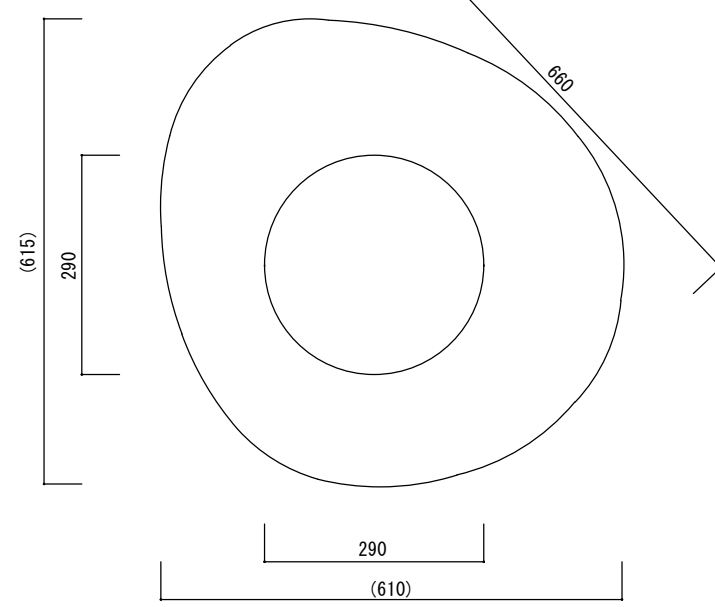
底面図
