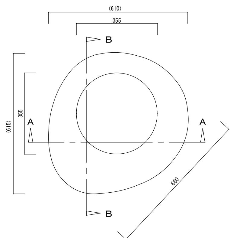
平面図
