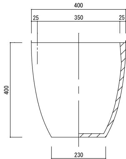
立・断面図
