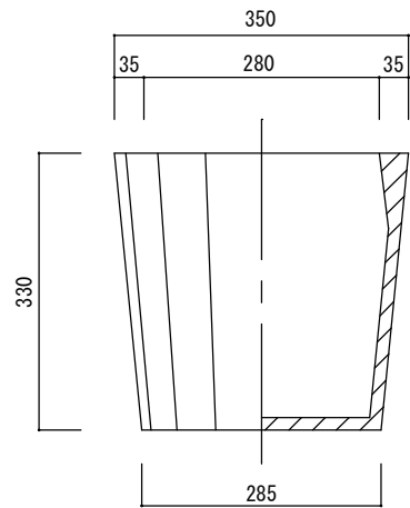
立・断面図
