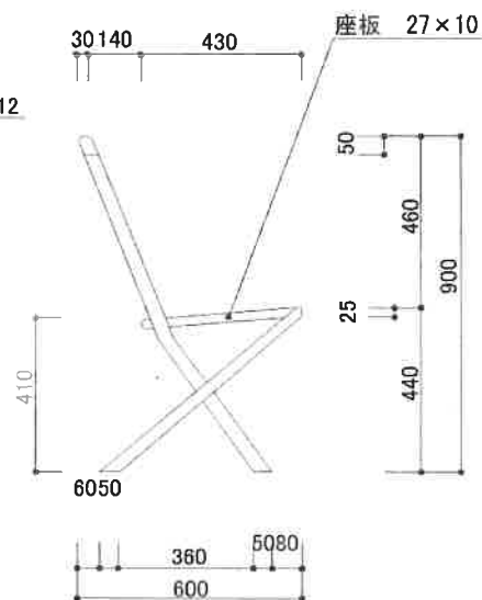
側面図
