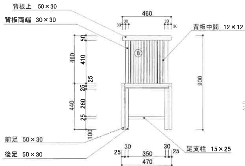
立面図
