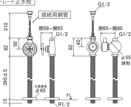
ストレート止水栓
