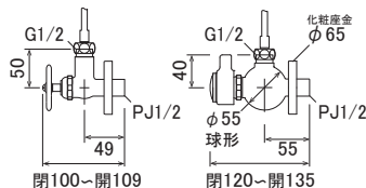
アングル止水栓
