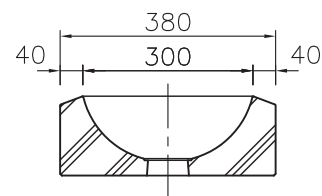
B-B断面図
