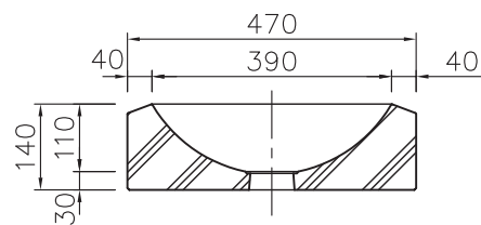
A-A断面図
