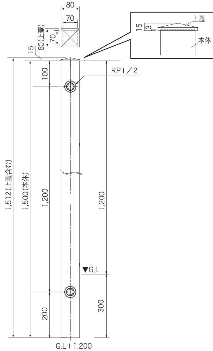
AL-150 〈正面図〉
