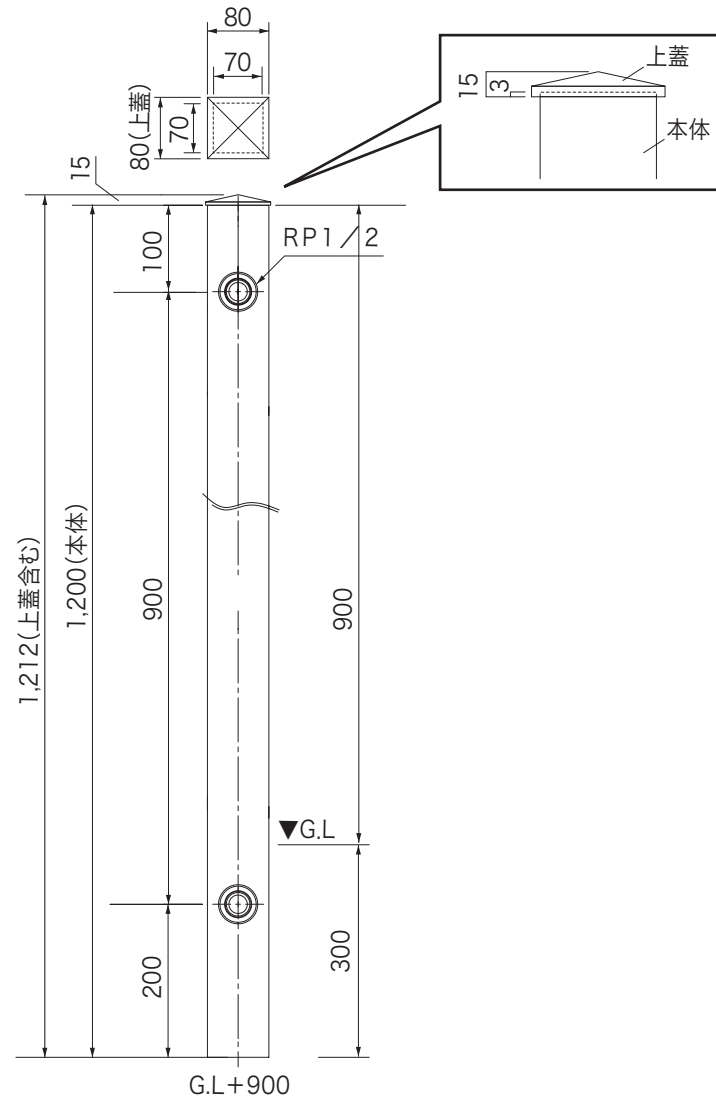
AL-100 〈正面図〉
