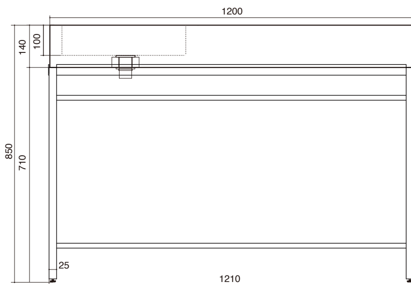
〈正面〉
