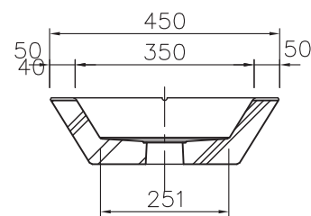
B-B断面図
