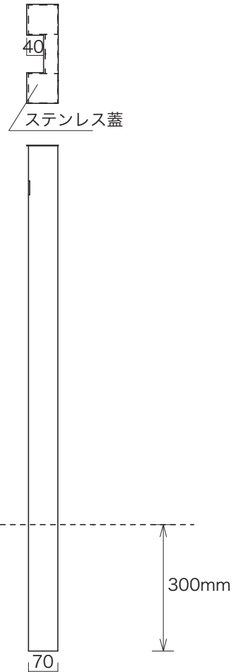
〈側面図〉
