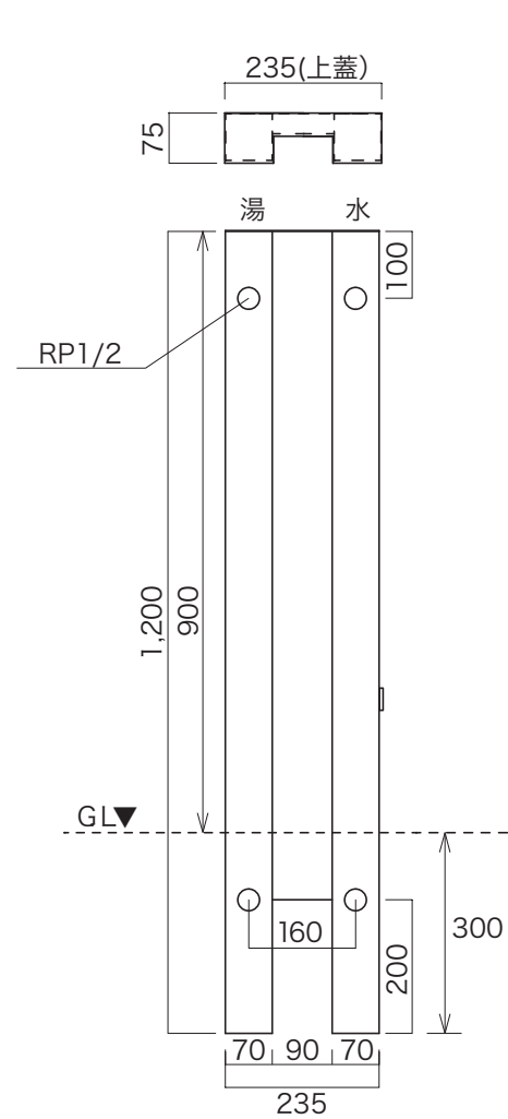
〈正面図〉
