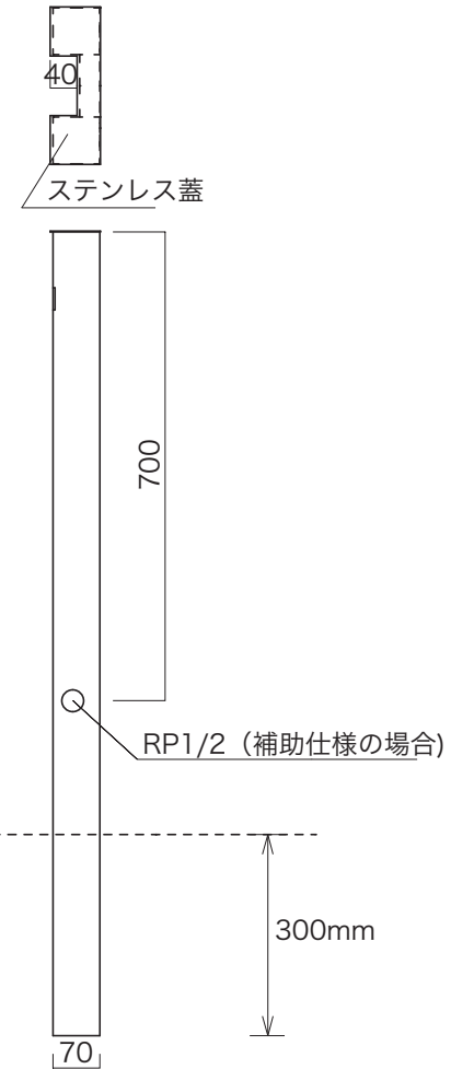
〈側面図〉
