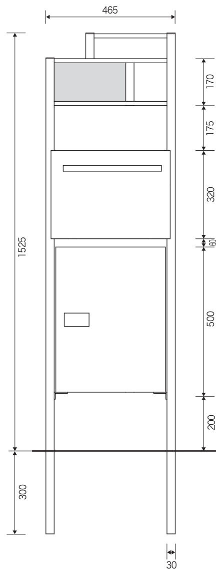
〈本体正面図〉
