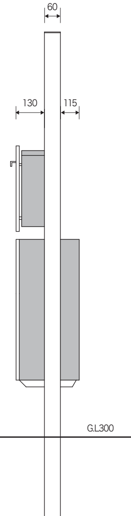
〈本体側面図ポストセット〉
