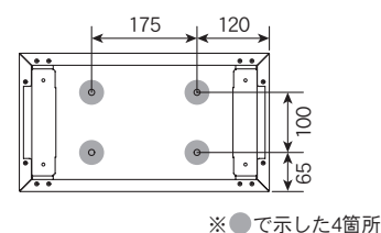
3 台座上面図 (アンカー用下穴位置)
