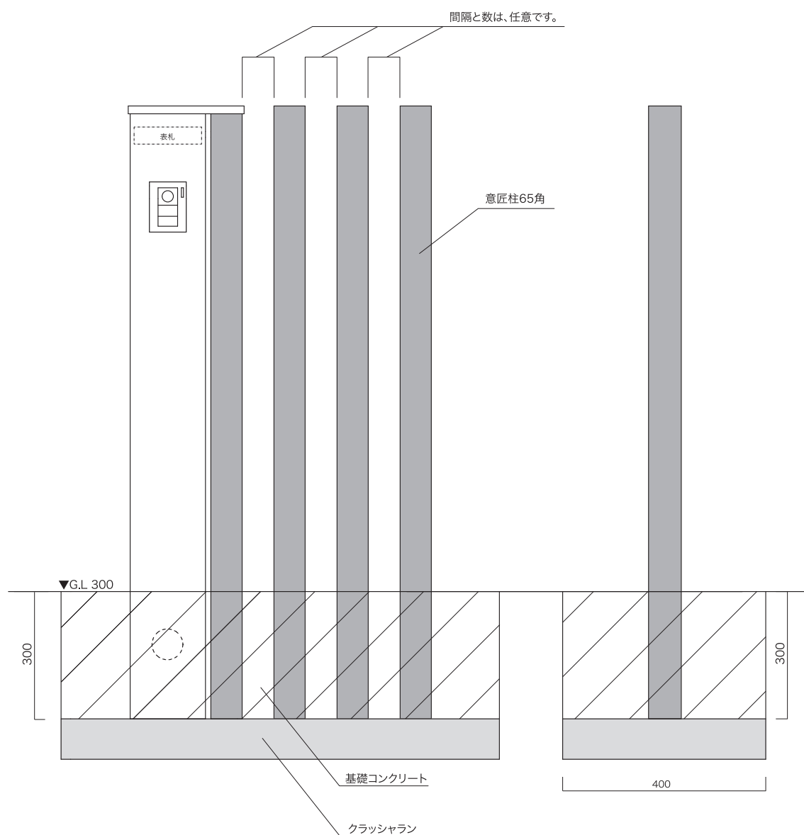
[正面図]
