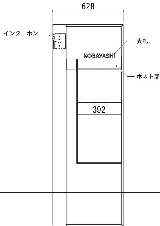
W628[2B]タイプ
