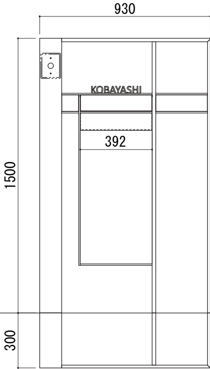
W930[1B]タイプ
