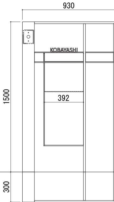
W930[2B]タイプ
