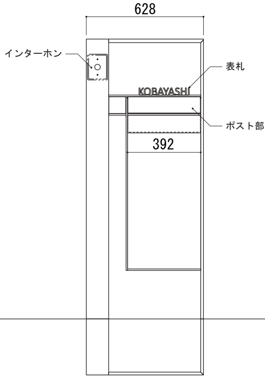
W628[1B]タイプ
