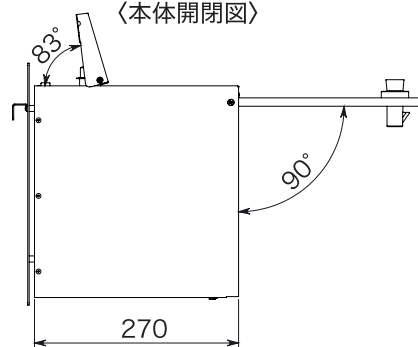
〈本体開閉図〉
