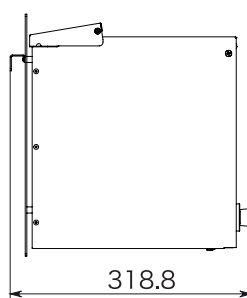
〈本体側面図〉
